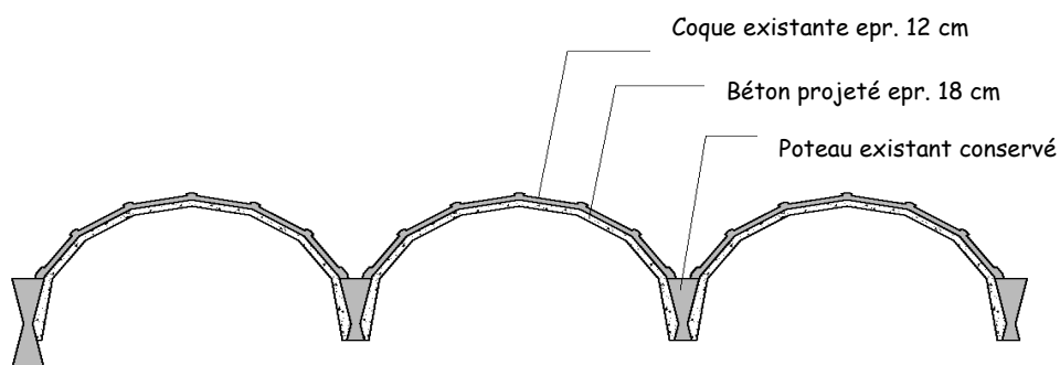
Partie Salle de spectacles - Renforcement des coques
