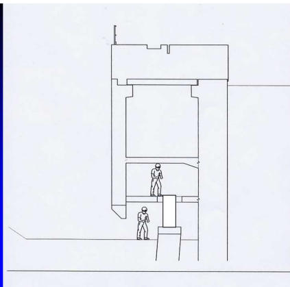
240m de réparation Poutre de Couronnement
