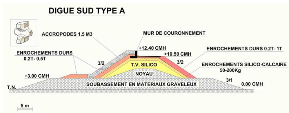
Coupe Type des digues
