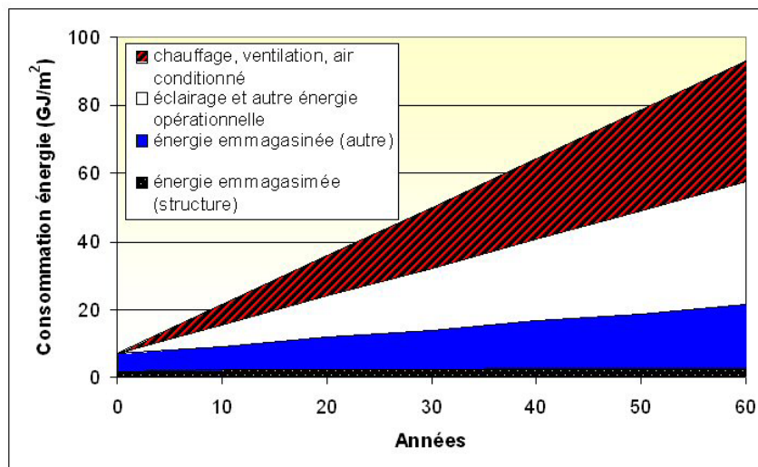
Figure 4: Energie emmagasinée et opérationnelle pour un bâtiment commercial avec une durée de vie de 60 ans
