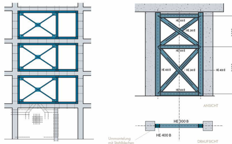
Figure 8: Exemple d'un renforcement sismique d'une structure historique à l'aide de cadres métalliques
