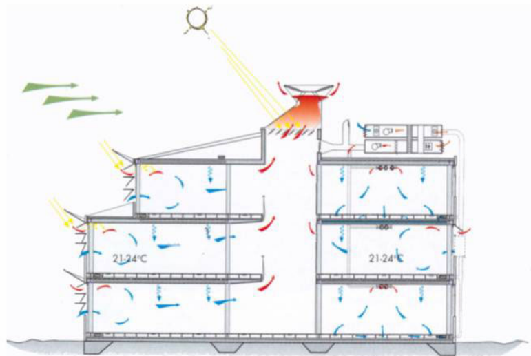
Figure 6: Bâtiment avec structure en acier et plancher conventionnels permettant une stratégie de ventilation naturelle
