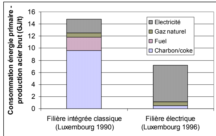
Figure 10: Comparaison de la consommation en énergie primaire des filières de production acier intégrée classique et électrique
