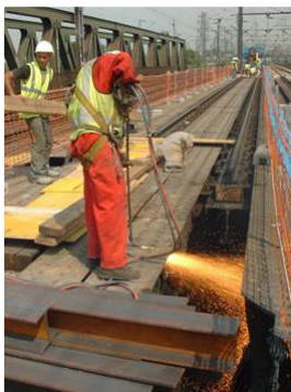
Découpe et évacuation du tablier ancien par dessous au milieu des circulations ferroviaires
