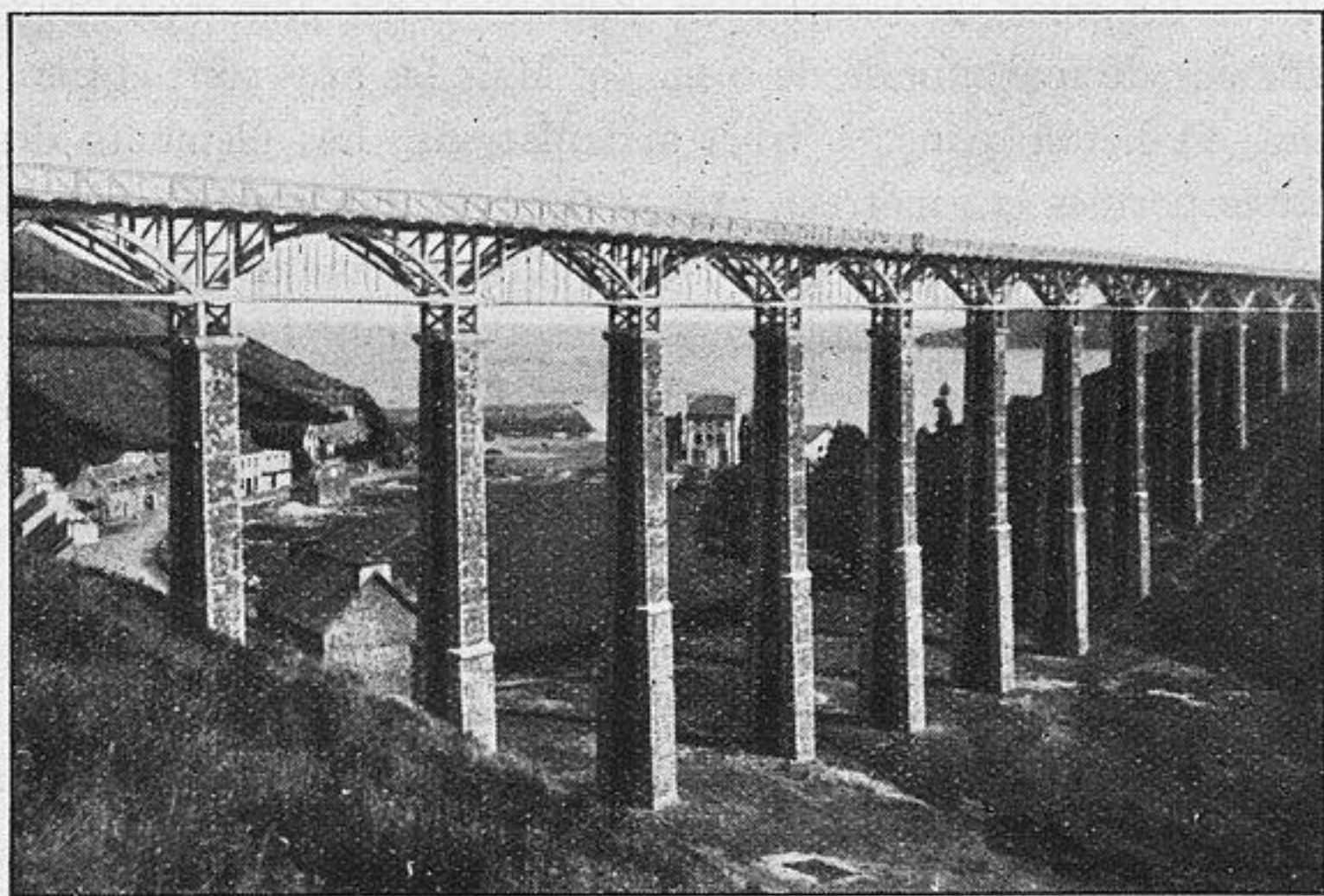
Fig. 7. — Ligné de Plouha à Paimpol. — Viaduc de Brehec (construit en 1913-1914). Longueur, 225 mètres ; hauteur, 32 m. 05 ; largeur, 4 m. 40. Travées de 12 mètres, arcs à 3 articulations. Piles oscillantes, palées en béton armé. Piles en maçonnerie à double T, avec tranches armées tous les deux mètres.
