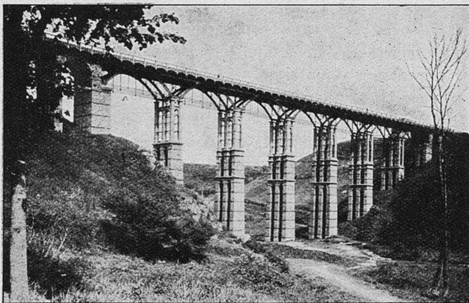
Fig. 2. — Ligne de Saint-Brieuc à Moncontour. — Viaduc de Toupin (construit en 1904). Longueur, 142 mètres hauteur, 44 mètres ; largeur 10 mètres. Piles en maçonnerie, en double T (à la base). Piliers briques et béton. Contreventement métallique. Arcs métalliques avec poutres raidissantes en béton armé.
