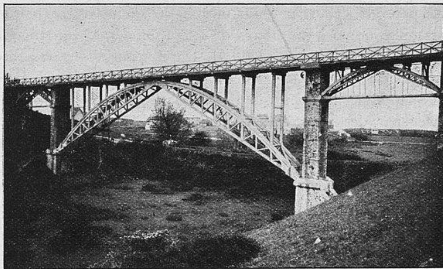
Fig. 6. — Ligne d'Yffiniac à Matignon. — Viaduc d'Erquy (construit en 1913-1914). Longueur, 80 mètres ; hauteur, 16 m. 20 ; largeur, 4 m. 40. Arc central de 45 mètres à trois articulations. Ouvrages d'approche. 2 travées de 12 mètres (arcs à 3 articulations).
