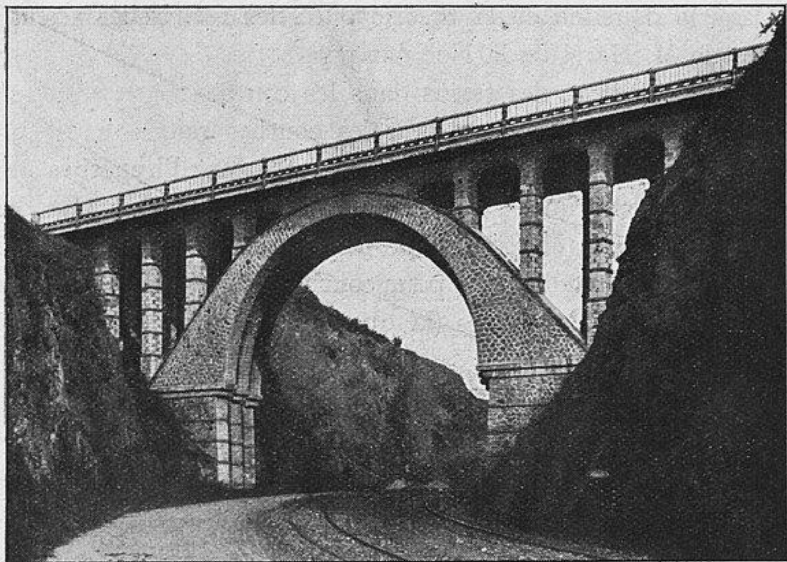
Fig. 3. — Ligne de Saint-Brieuc à Plouha. — Pont de Rohannet (construit en 1905). Pont biais, constitué par trois rouleaux en maçonnerie de 0 m. 70 de largeur, ouverture 20 mètres. Piliers en maçonnerie. Tablier en béton armé.
