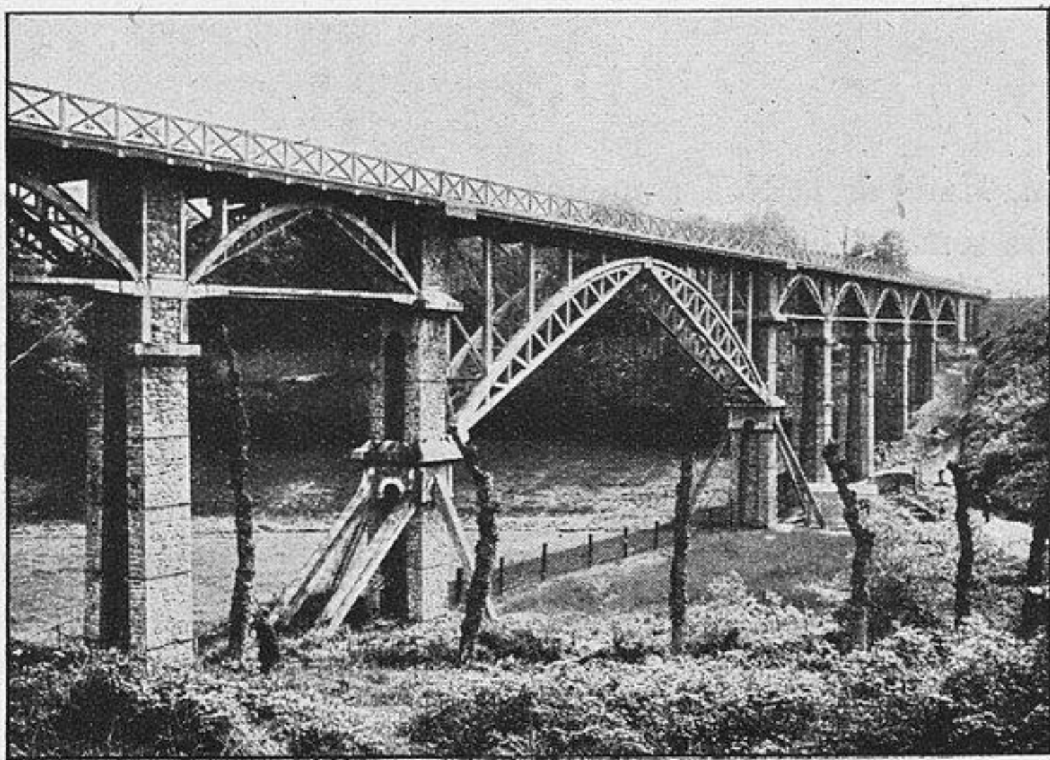
Fig. 8. — Ligne de Guingamp à Bourbriac. — Viaduc de Cadolan (construit en 1914-1915). Longueur totale, 205 mètres ; hauteur, 17 m. 65 ; largeur, 4 m. 40. Travée centrale. Arc à 3 articulations de 39 mètres. Travées latérales de 12 mètres. Arcs en béton armé à 3 articulations.
