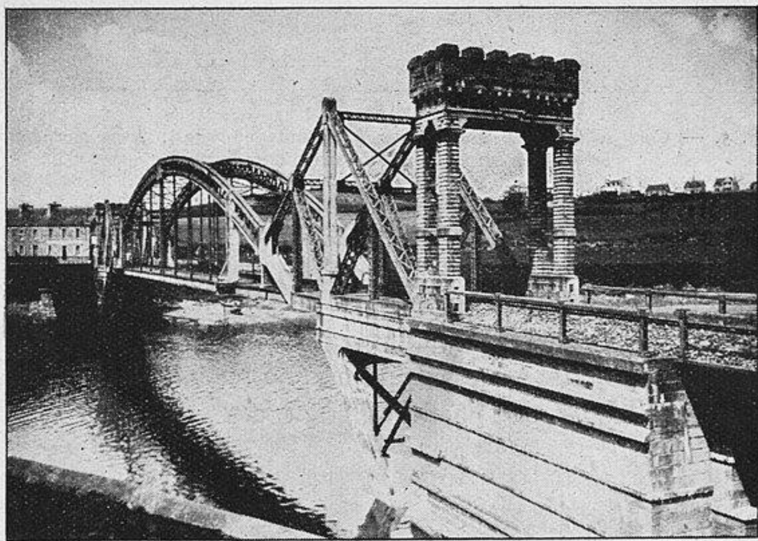
Fig. 4. — Ligne de Tréguier à Perros. — Pont sur le Guindy Maritime (construit en 1905-1906). Longueur totale, 190 mètres. Portée de 90 mètres entre culées. Arc en acier de 54 mètres de portée.
