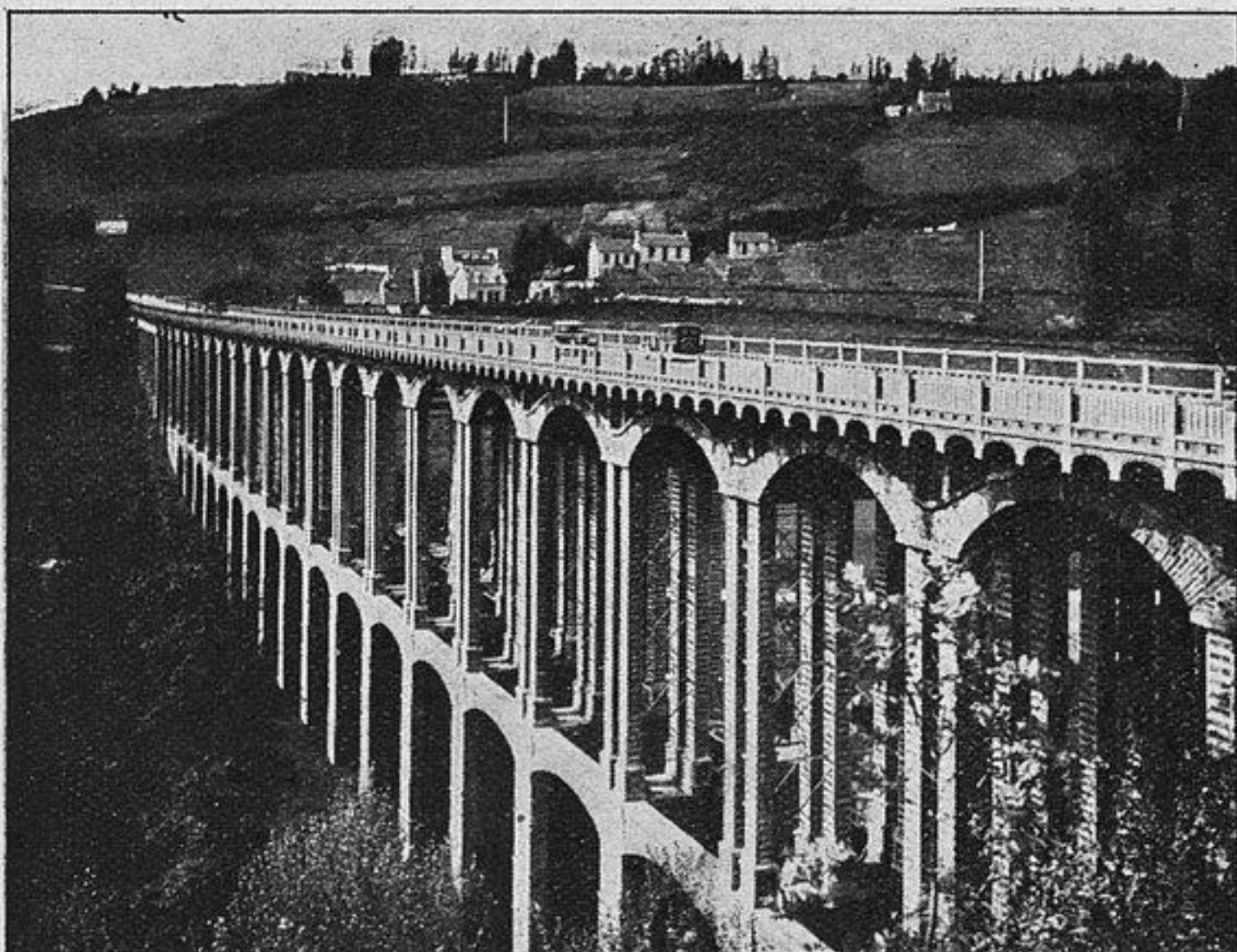
Fig. 1. — Ligne de Saint-Brieuc à Plouha. — Viaduc de Souzain (construit en 1904). Longueur, 280 mètres ; hauteur, 30 mètres ; largeur 13 mètres. Piles en double T (base), piliers, briques et béton (partie supérieure). — Rouleaux en maçonnerie en arcs surbaissés au cinquième, grands encorbellements.
