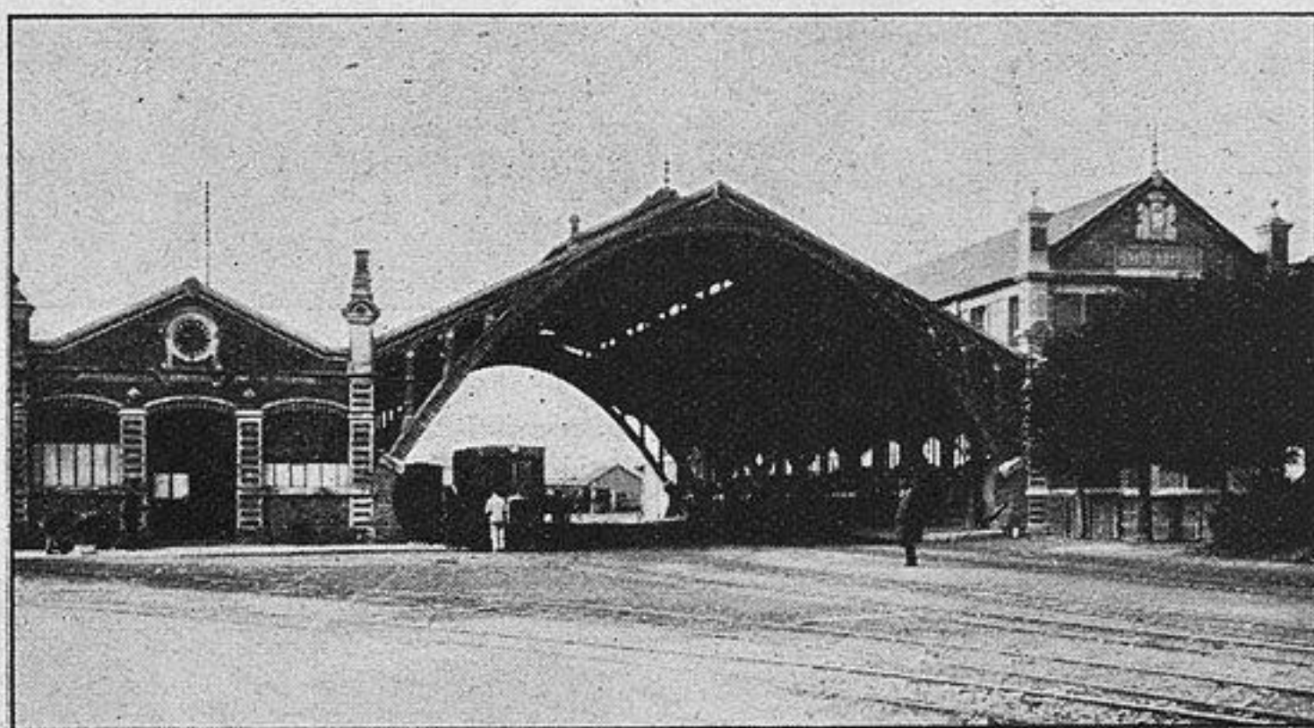
Fig. 5. — Gare centrale de Saint-Brieuc (construite en 1904). Avec parabolique briques et béton de 28 mètres d'ouverture.
